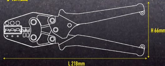
寸法図
